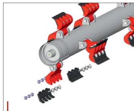
Schéma výměnných břitů u cepových mulčovačů
